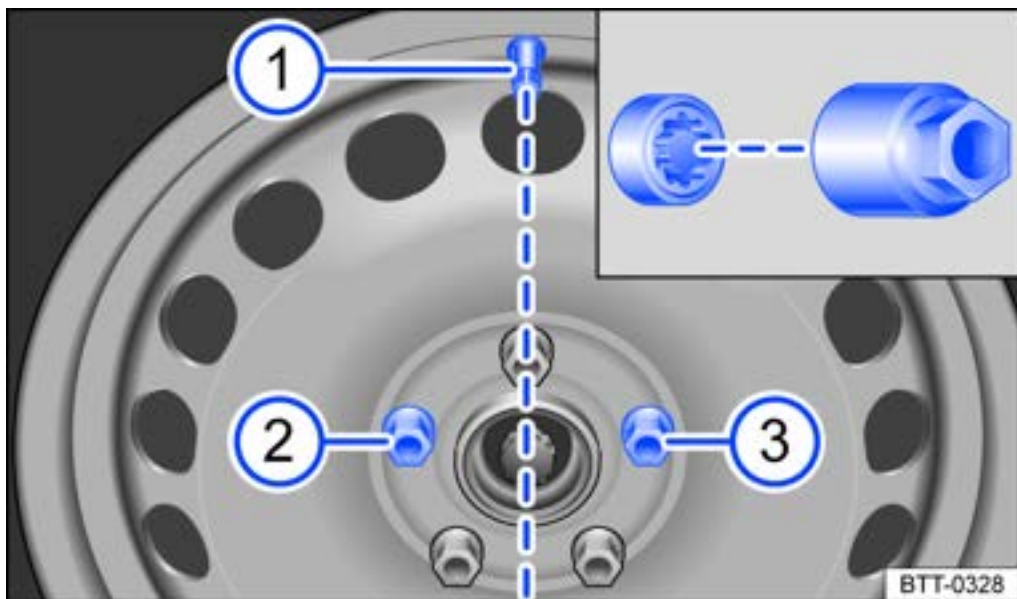
Abb. 2 Radwechsel: Reifenventil ① und Einbauorte der Anti-Diebstahl-Radschraube ② oder ③.
