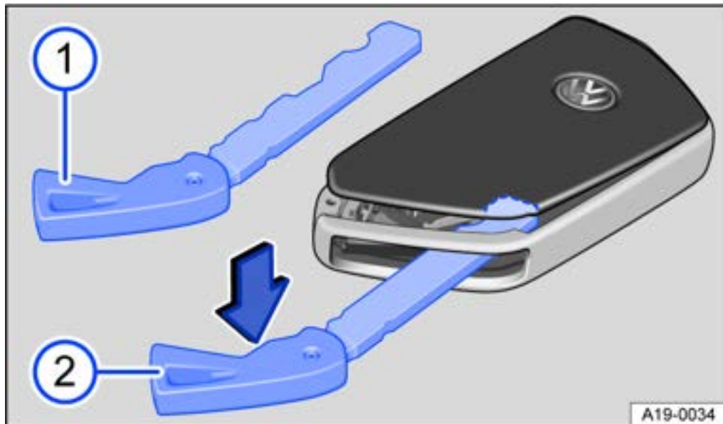
Abb. 1 Fahrzeugschlüssel: Batteriefachabdeckung öffnen.
