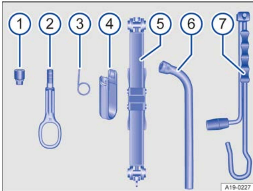
Abb. 1 Bestandteile des Bordwerkzeugs. (Prinzipdarstellung)
