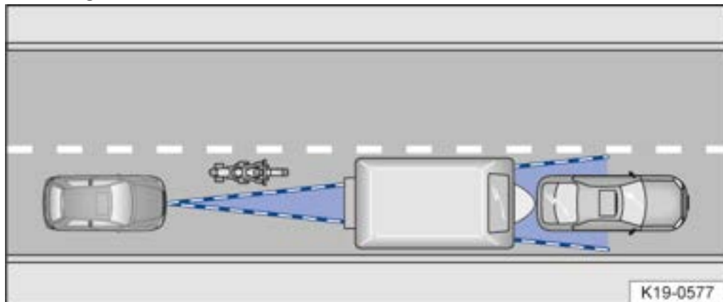
Abb. 3 Schmales Fahrzeug.
